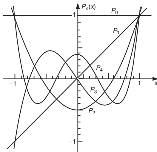
Fig. 4.5. Legendre polynomials
