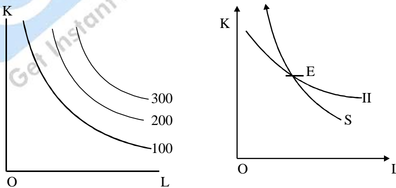
Fig. Isoquants
