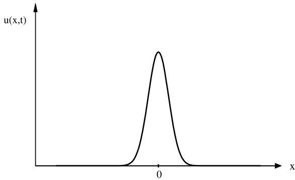
Fig. 9.15 A compacton.
