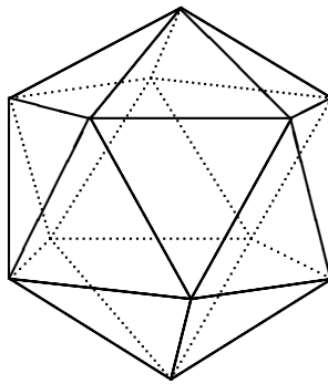
Fig. 6.6. Icosahedron.
