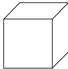
\{2, 3\} -residues cosets of \langle r_2, r_3 \rangle
